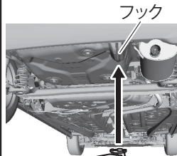
リヤ側ガレージジャッキ 指定位置(2WD車)
